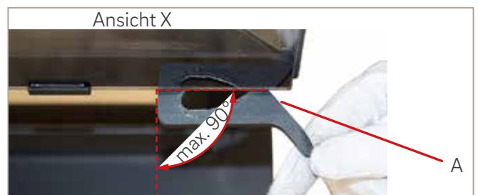
Abb. 45: „Verriegelungshebel unten“ bei 90 Grad geöffnet
